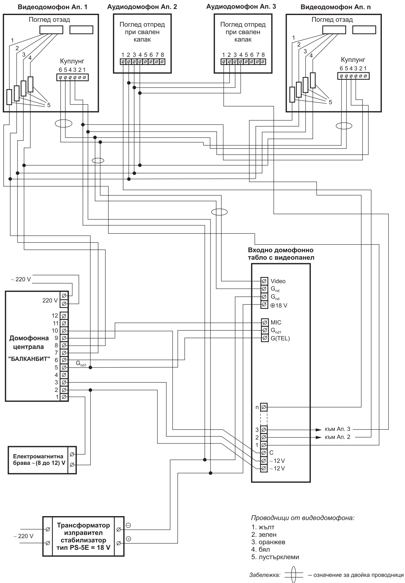
Схема на свързване на видеодомофонна система "БАЛКАНБИТ"
